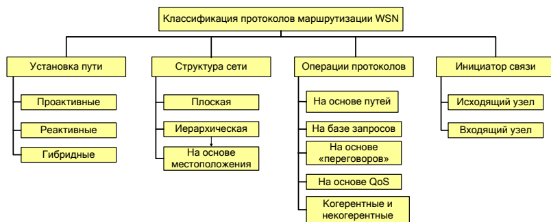
Рис. 3.10 – Классификация протоколов маршрутизации БСС
