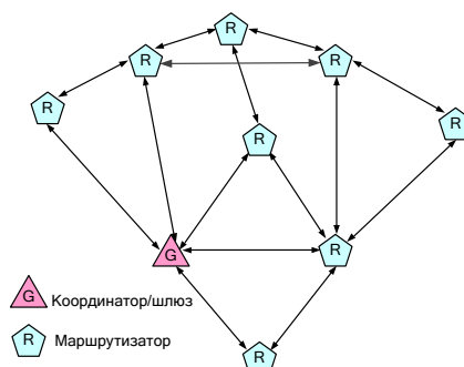
Рис. 3.8 – Ячеистая структура БСС
