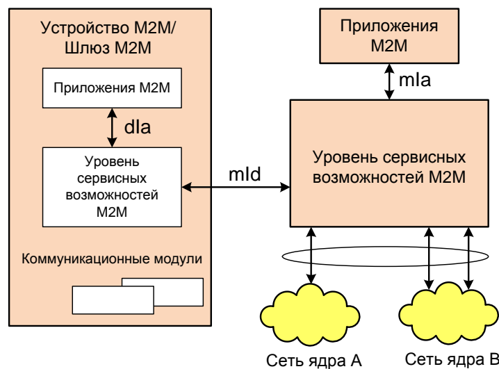
Рис. 4.3 – Интерфейсные точки функциональной архитектуры M2M (источник: ETSI)
